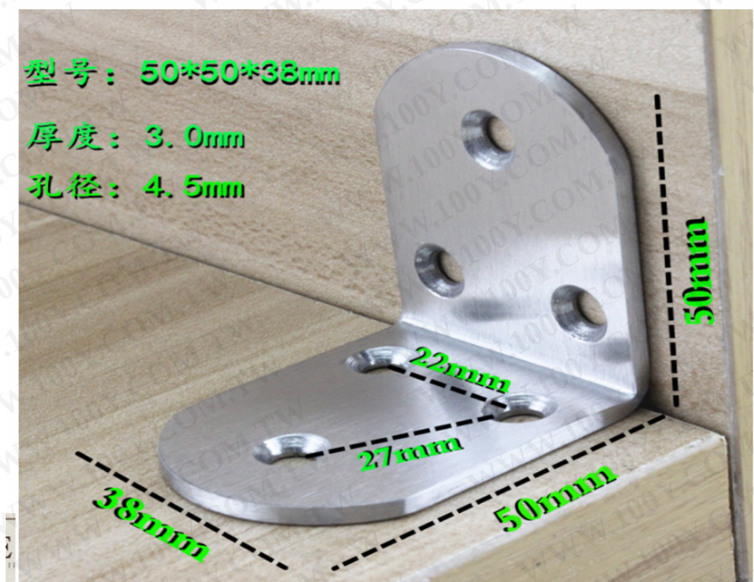
长50*长50*宽38*厚3mm规格尺寸图
